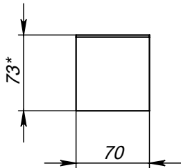
Поз.5 (Хомут)
