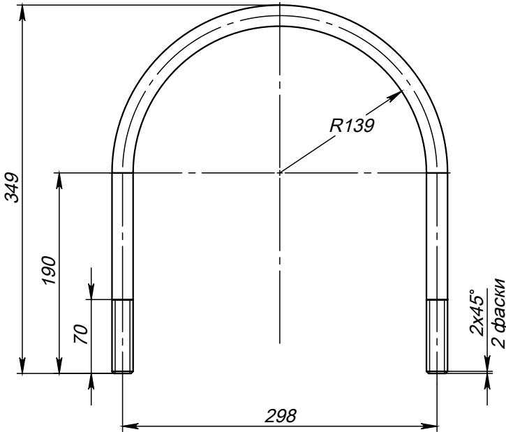
Поз.5 (Хомут)
